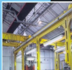
TRANSPORTADOR AÉREO COM CONJUNTO DE VENTILADORES PARA RESFRIAMENTO DO FERRO ELÉTRICO APÓS LINHA DE TESTE
